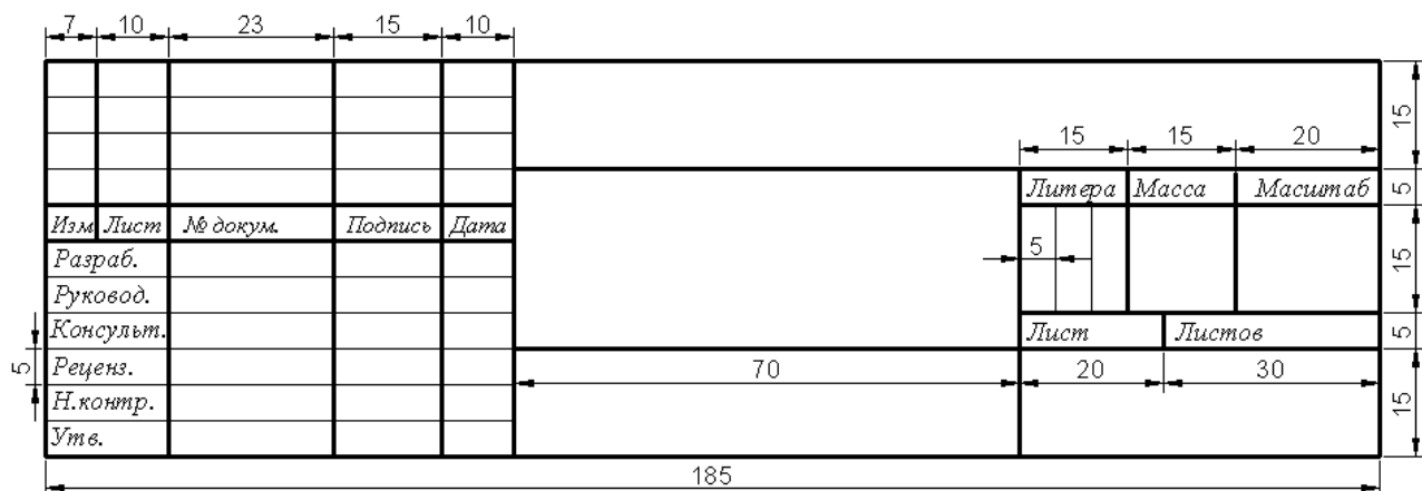
Рисунок 5 – Размеры основной надписи графической части
