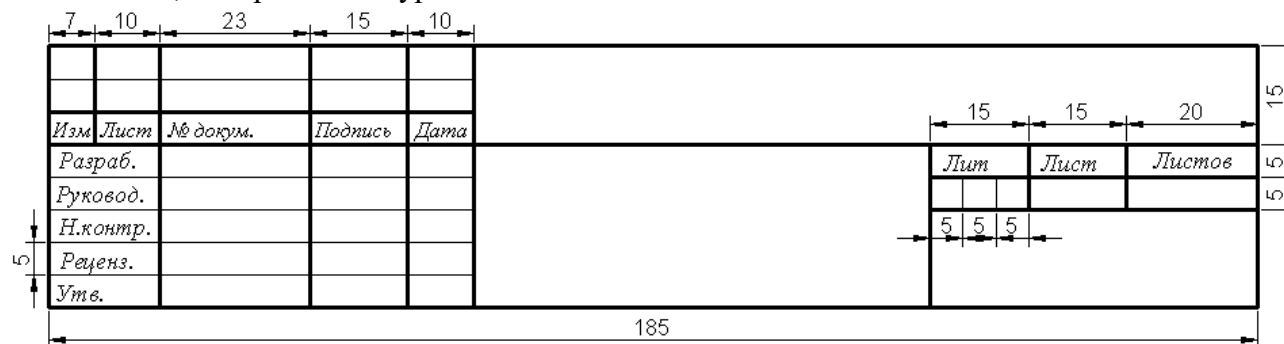
Рисунок 1 – Размеры основной надписи разделов ВКР
